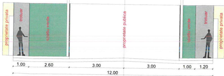
SECȚIUNE TRANSVERSALA STRADA PUBLICĂ PROPUȘĂ SC. 1:200
