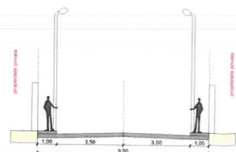
SECȚIUNE TRANSVERSALA STRADA PUBLICĂ PROPUȘĂ SC. 1:200
