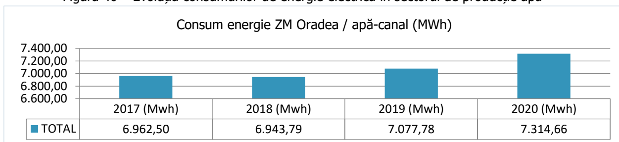
Figura 40 – Evoluția consumurilor de energie electrică în sectorul de producție apă
