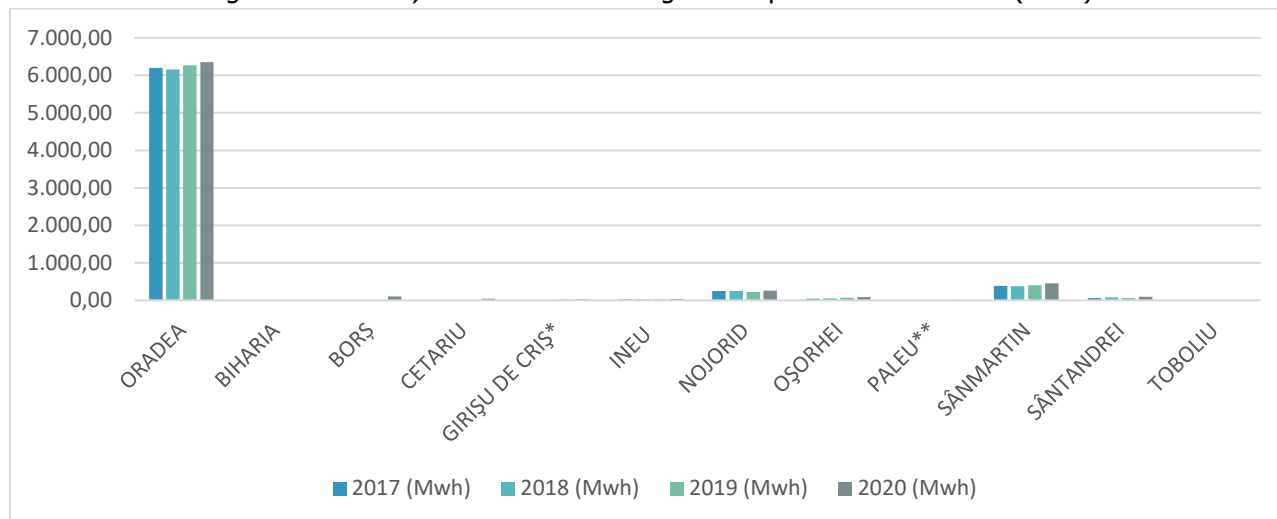
Figura 39 – Evoluția consumurilor energetice în perioada 2017-2020 (MWh)
